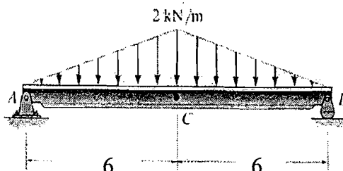
圖二 梁
